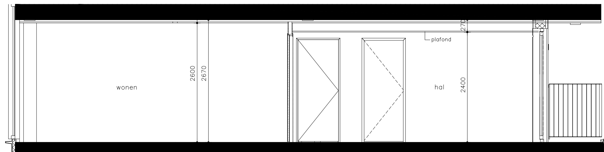
Doorsnede
